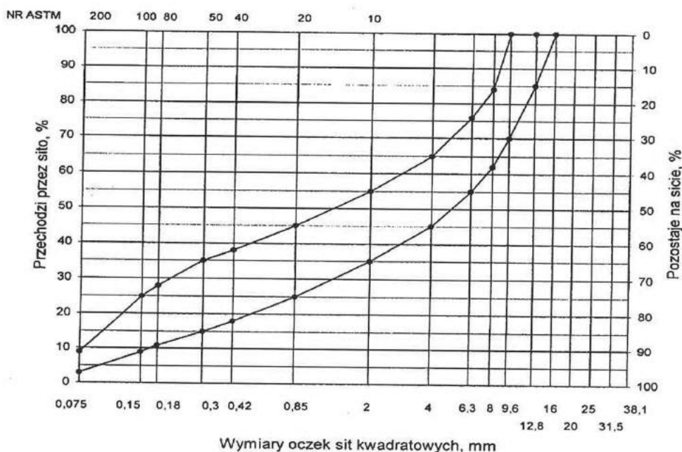
Rys. 6. Krzywe graniczne uziarnienia mieszanki mineralnej BA od 0 do 12,8 mm do warstwy wiążącej, wyrównawczej i wzmacniającej nawierzchni drogi o obciążeniu ruchem KR1 i KR2
