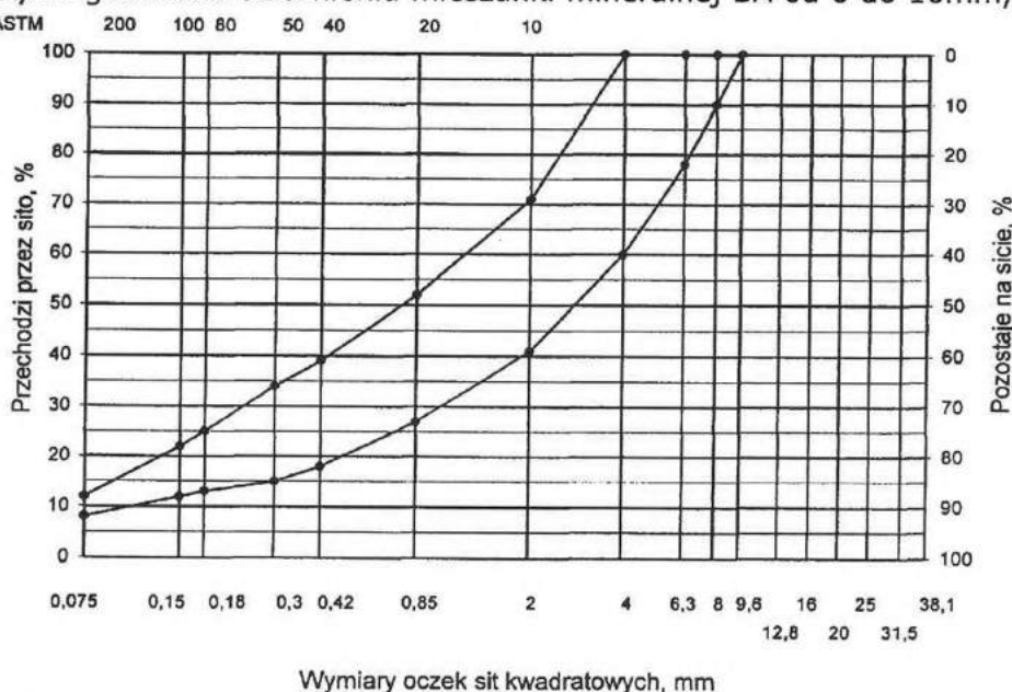
Rys. 3. Krzywe graniczne uziarnienia mieszanki mineralnej BA od 0 do 8mm, od 0 do 6,3 mm do warstwy ścieralnej nawierzchni drogi o obciążeniu ruchem KR1 i KR2
