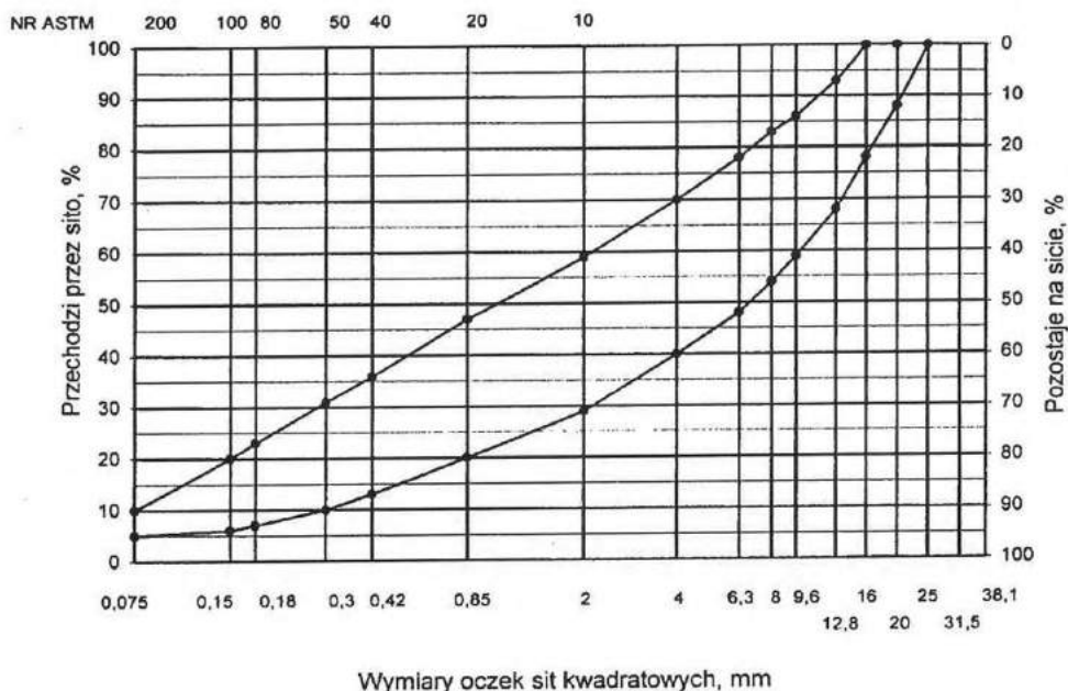
Rys. 1. Krzywe graniczne uziarnienia mieszanki mineralnej BA od 0 do 20 mm do warstwy ścieralnej nawierzchni drogi o obciążeniu ruchem dla KR1 i KR2
