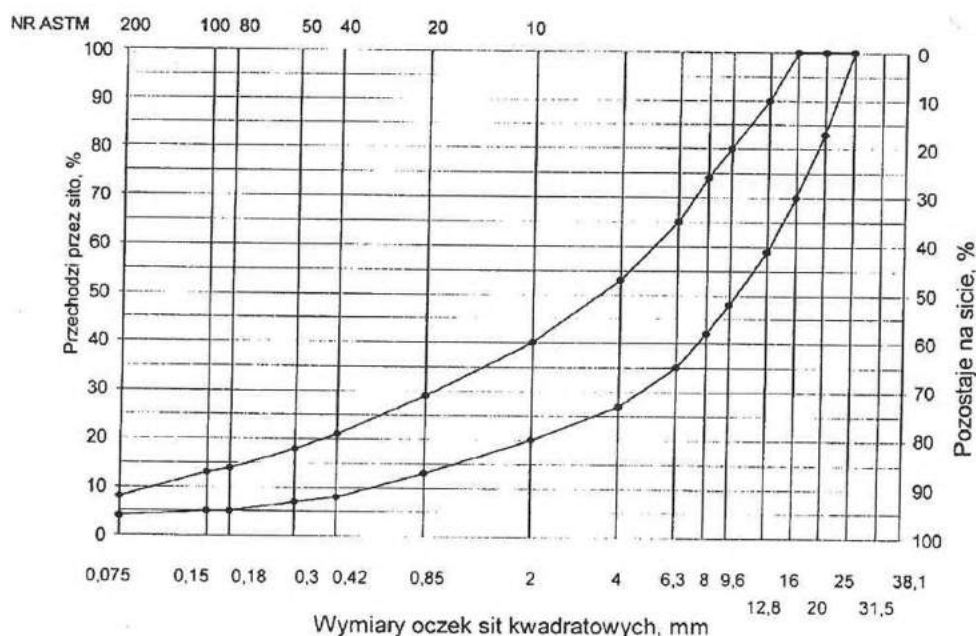
Rys. 3. Krzywe graniczne uziarnienia mieszanki mineralnej BA od 0 do 20 mm do podbudowy nawierzchni drogi o obciążeniu ruchem KR 1, 2
