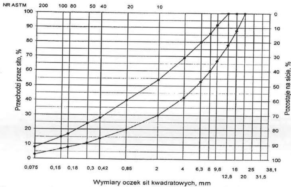
Rys. 5. Krzywe graniczne uziarnienia mieszanki mineralnej BA od 0 do 16 mm do warstwy wiążącej, wyrównawczej i wzmacniającej nawierzchni drogi o obciążeniu ruchem KR1 i KR2
