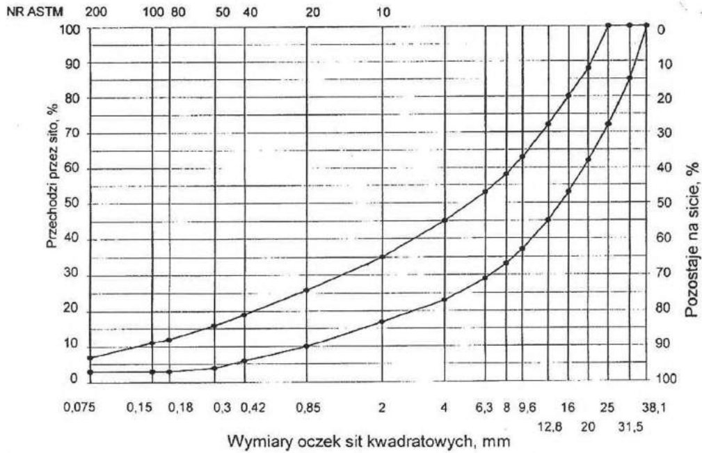
Rys.1. Krzywe graniczne uziarnienia mieszanki mineralnej BA od 0 do 31,5 mm do podbudowy nawierzchni drogi o obciążeniu ruchem KR 1, 2
