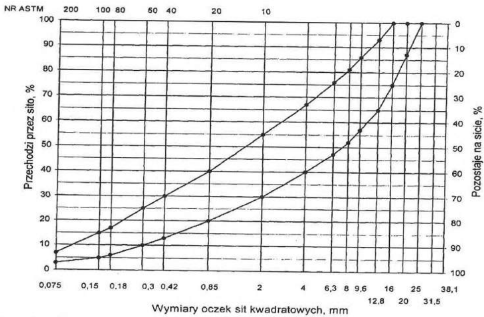
Rys. 4. Krzywe graniczne uziarnienia mieszanki mineralnej BA od 0 do 20 mm do warstwy wiążącej, wyrównawczej i wzmacniającej nawierzchni drogi o obciążeniu ruchem KR1 i KR2
