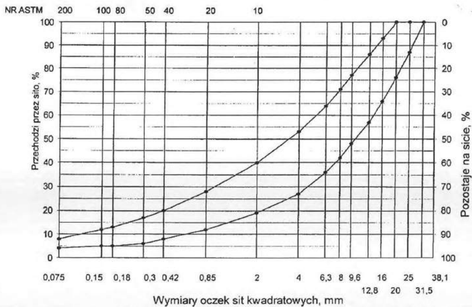
Rys. 2. Krzywe graniczne uziarnienia mieszanki mineralnej BA od 0 do 25mm do podbudowy nawierzchni drogi o obciążeniu ruchem KR 1, 2
